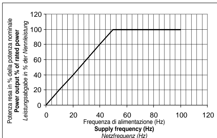
Fig. 2 - Diagramma potenza resa - frequenza
